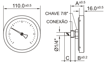
Modelo FTI-100/2 100 mm
