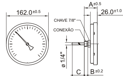
Modelo FTI-160/2 160 mm
