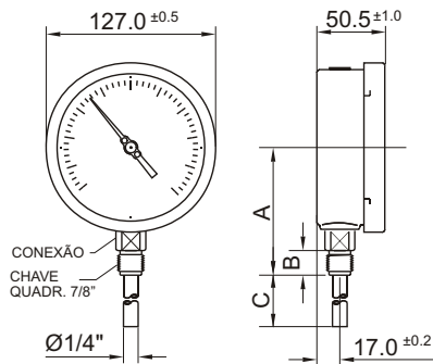
Modelo FTI-114/1 114 mm
