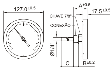
Modelo FTI-114/2 114 mm
