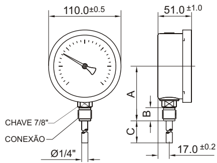
Modelo FTI-100/1 100 mm
