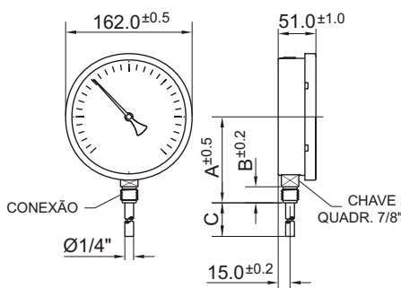
Modelo FTI-160/1 160 mm
