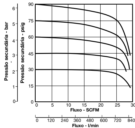
Mola de alta pressão - 0 a 8,5 bar
