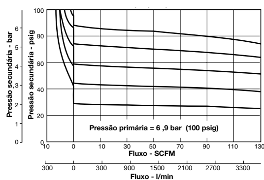
Rosca de 1/2"
