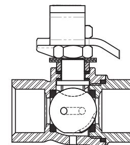
DETALHE PARA VÁLVULA COM FURO DE ALÍVIO DE PRESSÃO
