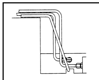
Montagem incorreta
