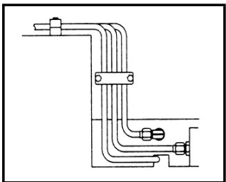
Montagem correta
