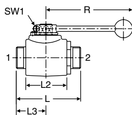
Diâmetro nominal 32 - 40
