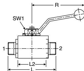
Diâmetro nominal 4 - 25
