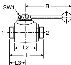
Diâmetro nominal 32 - 40
